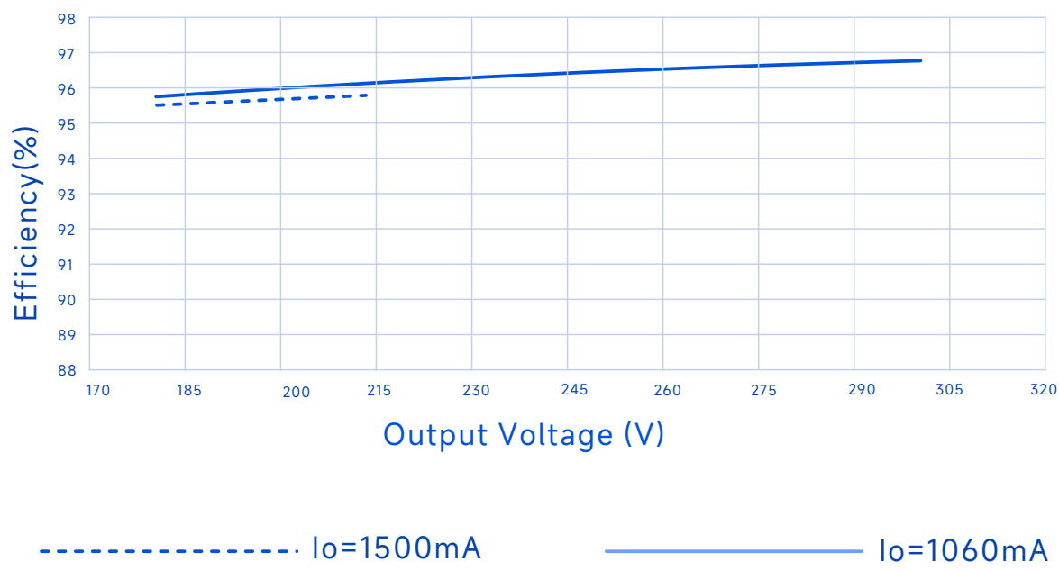
效率 Vs. 输出电压 (Vin=347Vac)
